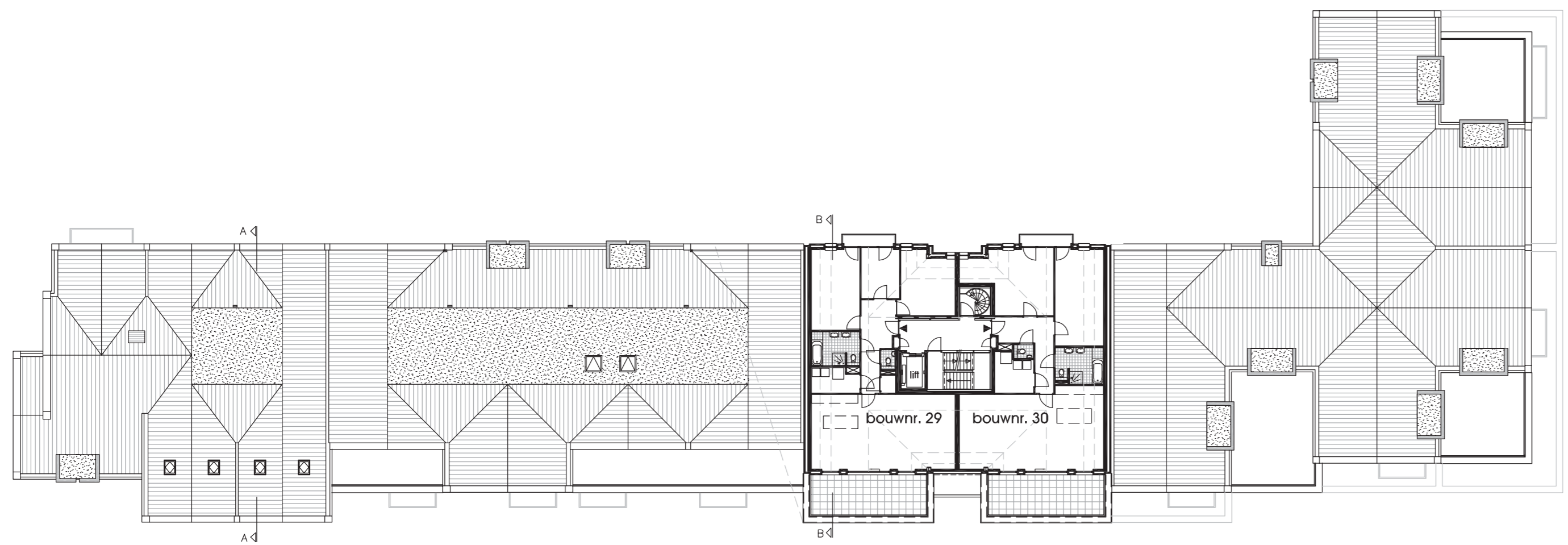
DERDE VERDIEPING
